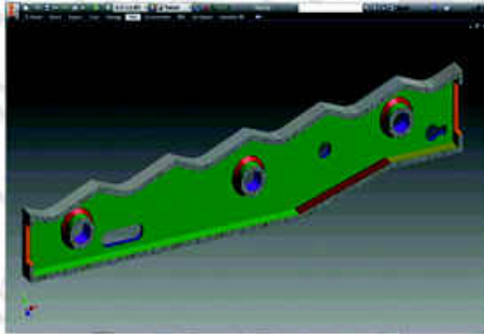
■ شانه ها و مقر شانه های کوره خط تولید نورد لوله Pipe Seat and Supports for Hot-rolled Pipe Production Line Furnace
